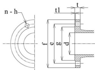
Flange DIN PN16
