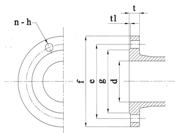
Flange DIN PN16
